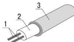
Рисунок 4.3 – Конструкция ЧЭ на основе КТМС
